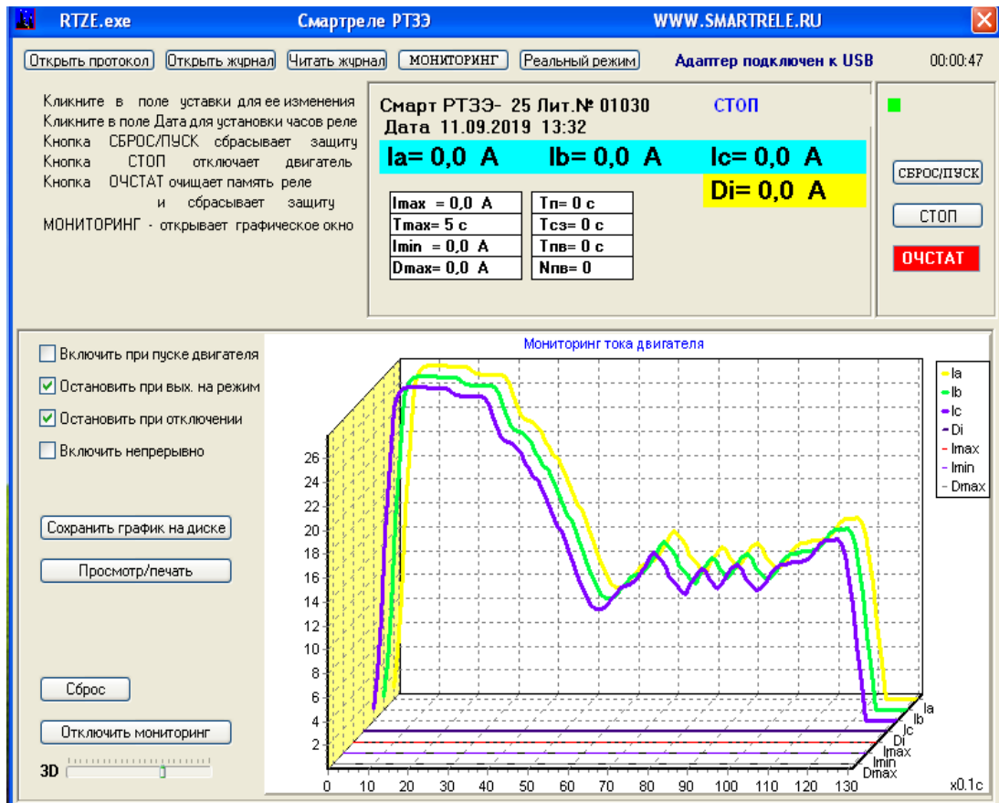
Рисунок 7 - отображение мониторинга работы двигателя, оснащенного Смартреле PT33, в реальном времени
