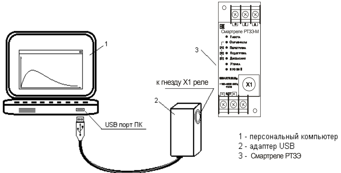
Рисунок 6 – соединение Смартреле PT33 с ПК при помощи адаптера USB
