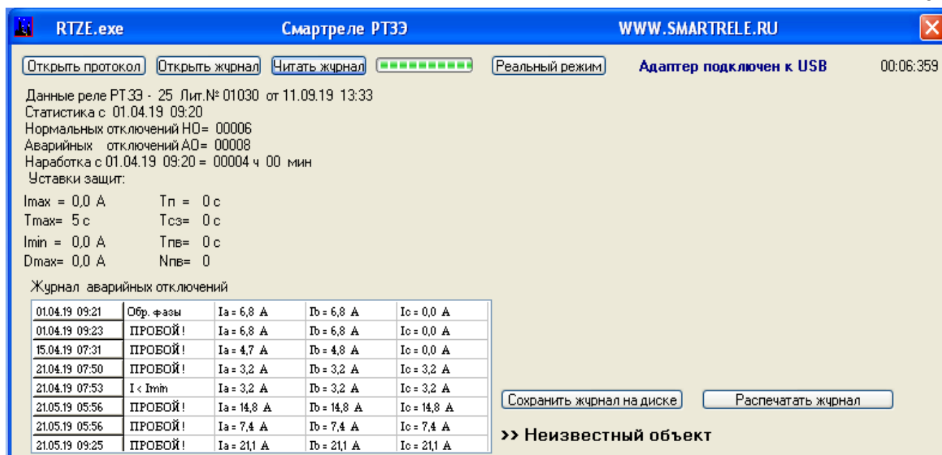
Рисунок 8 - отображение журнала событий Смартреле PT3Э на экране ПК
